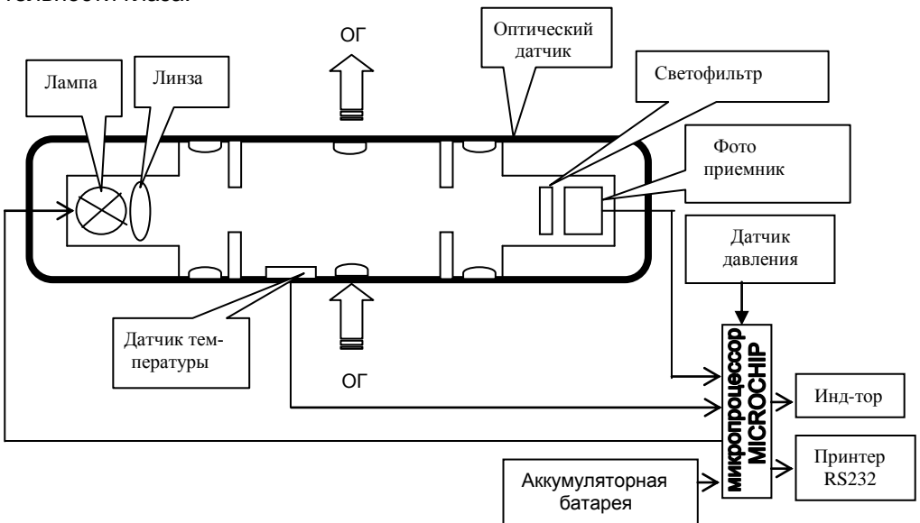
Рисунок 6 – Функциональная схема дымомерного канала
